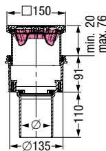
Afbeelding toont Art. Nr. 34 102 (verticale afvoer)
