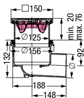
Afbeelding toont Art. Nr. 34 101 (zijwaartse afvoer)
