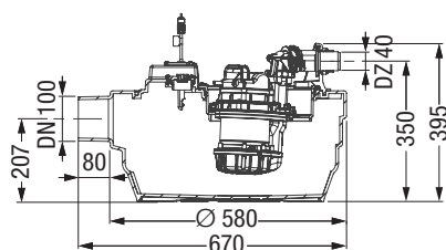
Rys.: urządzenie Mono 28 711-C
