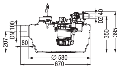
Rys.: urządzenie Duo 28 743-C
