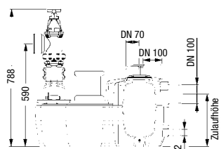
Abb.: Duoanlage
