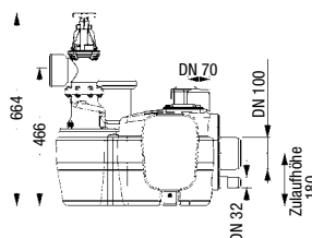
Abb.: Monoanlage
