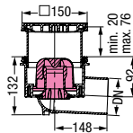
Abb.: Artikel 45 110.40 (Auslauf seitlich)
