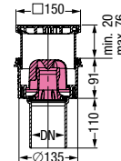
Abb.: Artikel 45 210.40 (Auslauf senkrecht)
