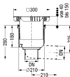
Abb.: Artikel 67 020.30, 67 060.30
